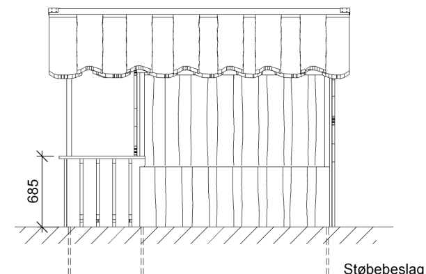
Sidebillede
